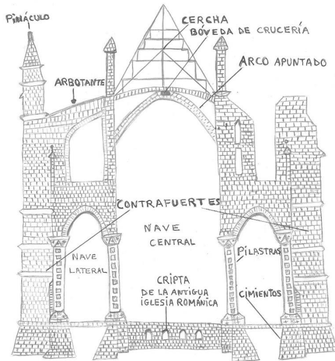
IGLESIA GÓTICA CORTE TRANSVERSAL ELEMENTOS ESTRUCTURALES
